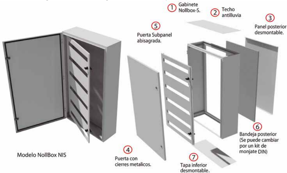
Figura 3. Partes del gabinete estanco para interiores Nöllbox-S
