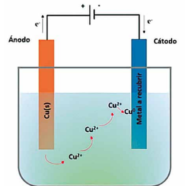
Figura 2. Cobreado
