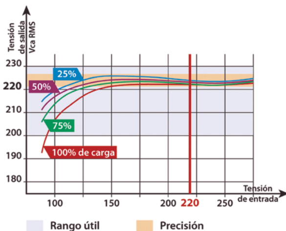
Comportamiento ferorrresonante
