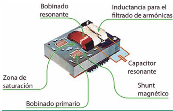
Esquema de un ferorrresonante
